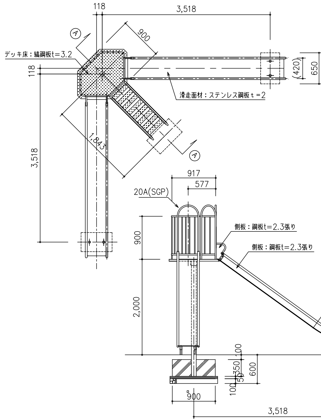
立面図 S=1/40
