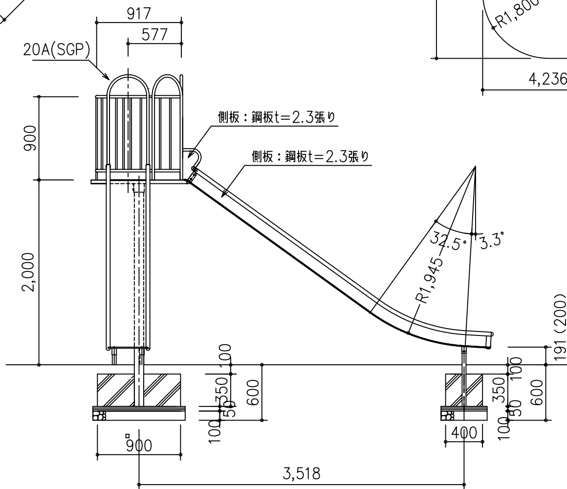
立面図 S=1/40
