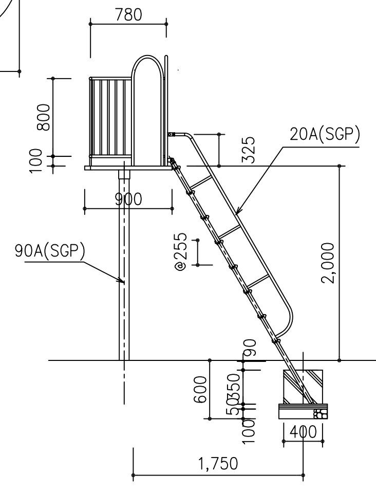
A-A矢視図 S=1/40
