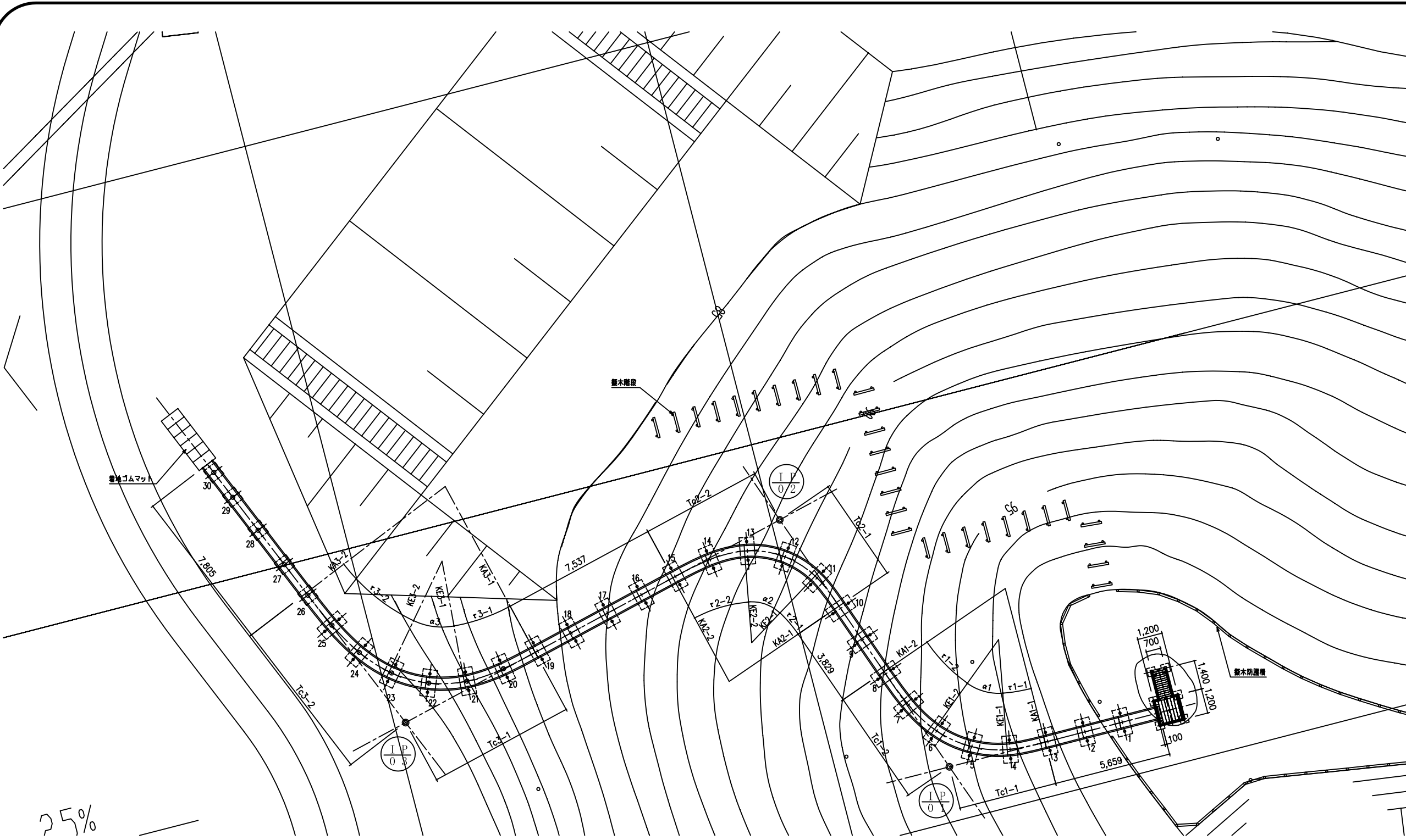
平面配置図
