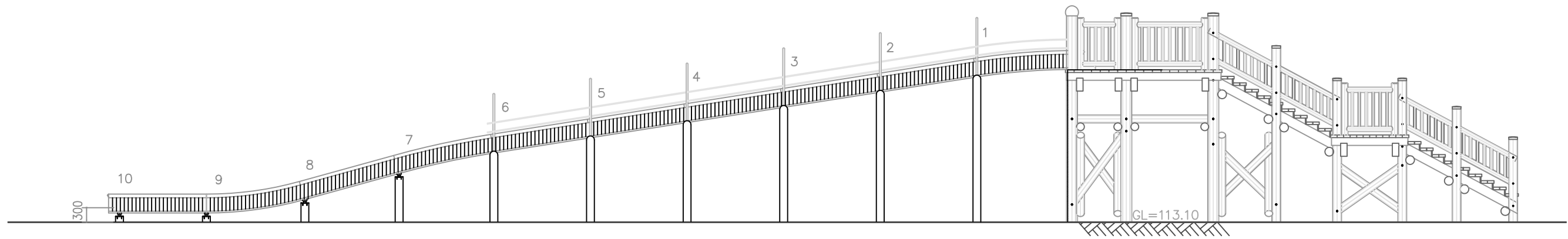
立面図 S=1/100
